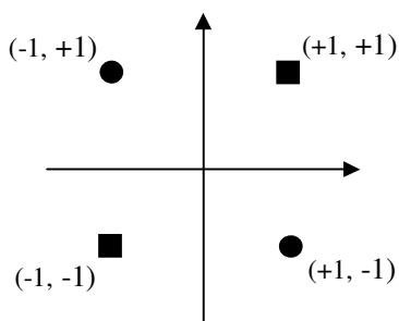
Figura A.2 – Conjunto de dados não linearmente separáveis do operador XOR.
