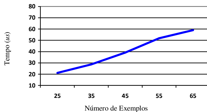
Figura 37 - Tempo necessário para a classificação utilizando a SVM do agente Diretor de Fotografia/Diretor de Música com bases de treinamento de tamanho variado.
