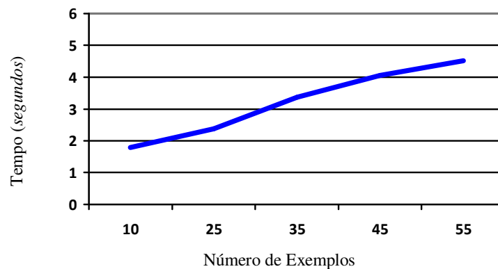
Figura 33 - Tempo necessário para o treinamento das 9 SVMs do agente Editor utilizando bases de treinamento de tamanho variado.
