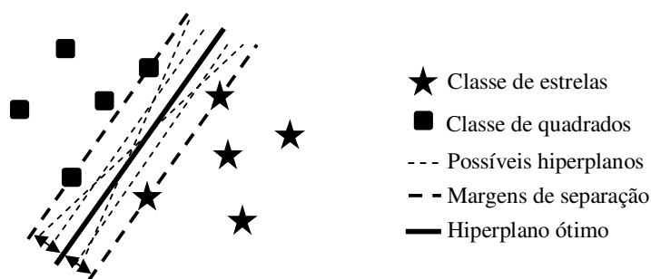
Figura A.1 - Hiperplano ótimo separando duas classes de dados.
