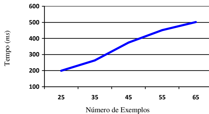
Figura 36 - Tempo necessário para o treinamento da SVM do agente Diretor de Fotografia/Diretor de Música utilizando bases de treinamento de tamanho variado.
