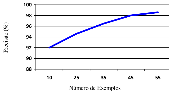
Figura 35 - Taxa de reconhecimento das SVMs do agente Editor utilizando bases de treinamento de tamanho variado.
