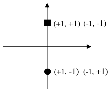
Figura A.3 – Problema do operador XOR no espaço de características transformado.
