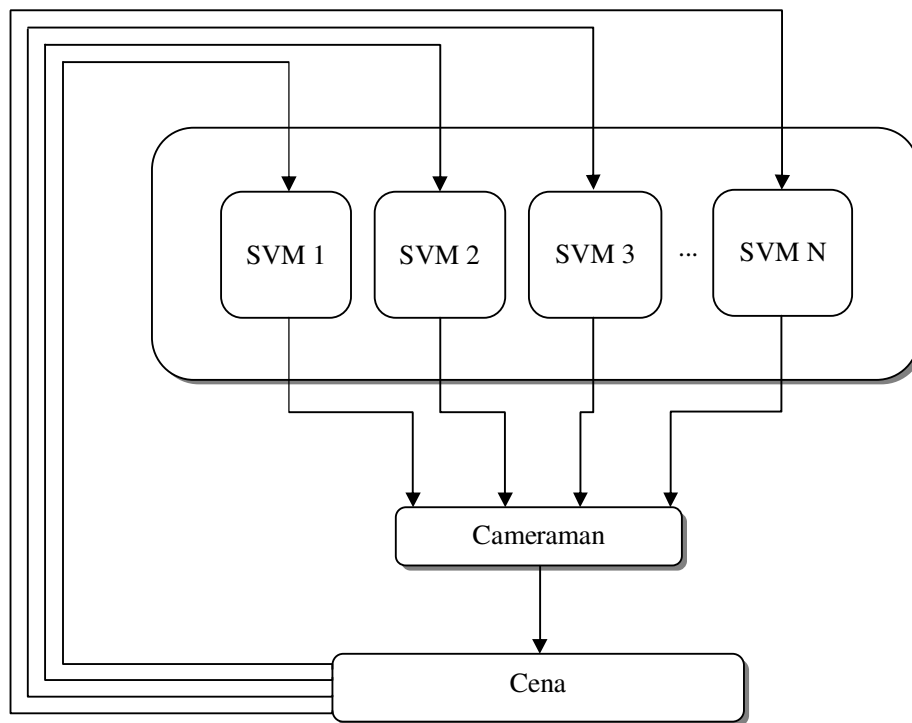
Figura 23 - Arquitetura do agente Editor.
