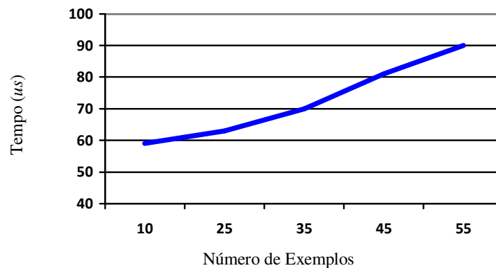
Figura 34 - Tempo necessário para a classificação utilizando as SVMs do agente Editor com bases de treinamento de tamanho variado.
