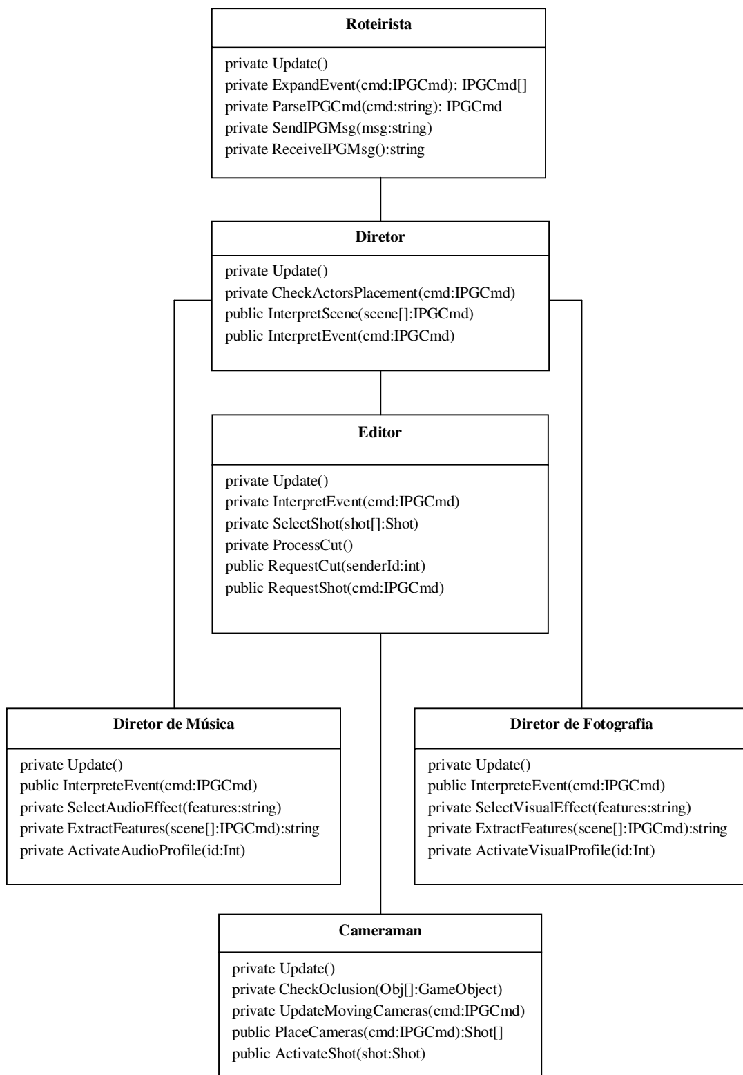
Figura 17 - Diagrama de classes dos agentes cinematográficos.
