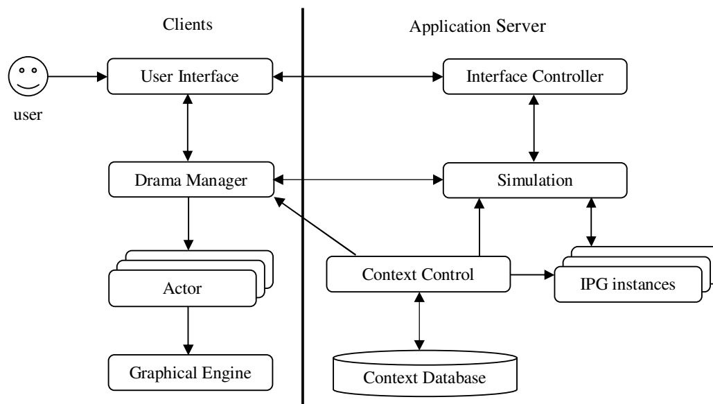
Figura 2 - Arquitetura do Logtell. Fonte: Camanho et al. (2009).
