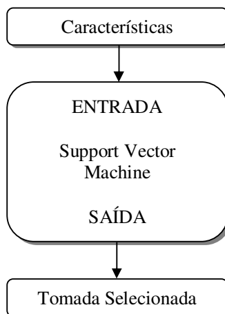
Figura 24 - Modelo de entrada, processamento e saída de dados das SVMs do agente Editor.
