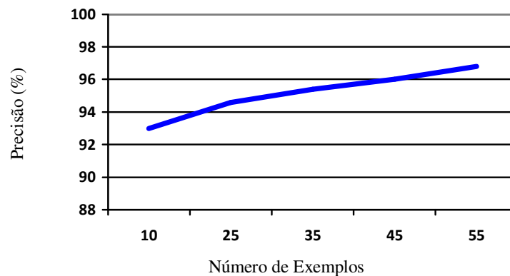
Figura 38 - Taxa de reconhecimento da SVM do agente Diretor de Fotografia/Diretor de Música utilizando bases de treinamento de tamanho variado.
