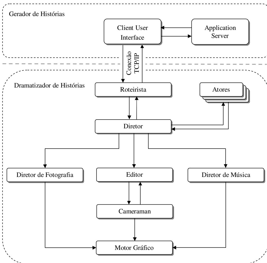
Figura 15 - Arquitetura de dramatização cinematográfica.
